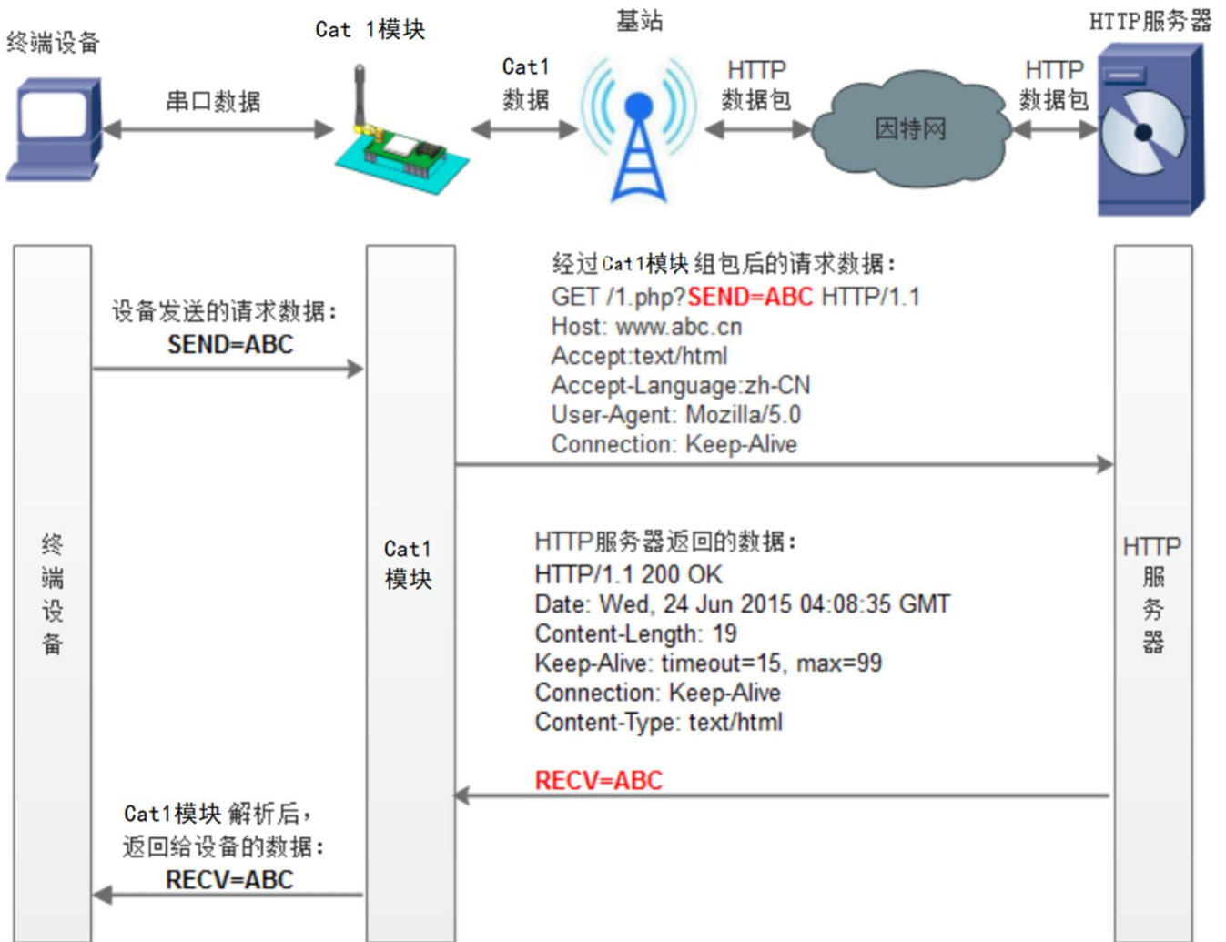
图 6. HTTPD Client 模式
