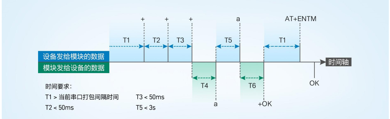
图 28. 切换指令模式时序
